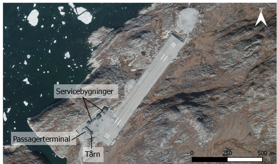
Takussutissiaq 3.1: Mittarfik pioreersoq tassunga ilaasut illuliat aamma atortorissaarutit.
