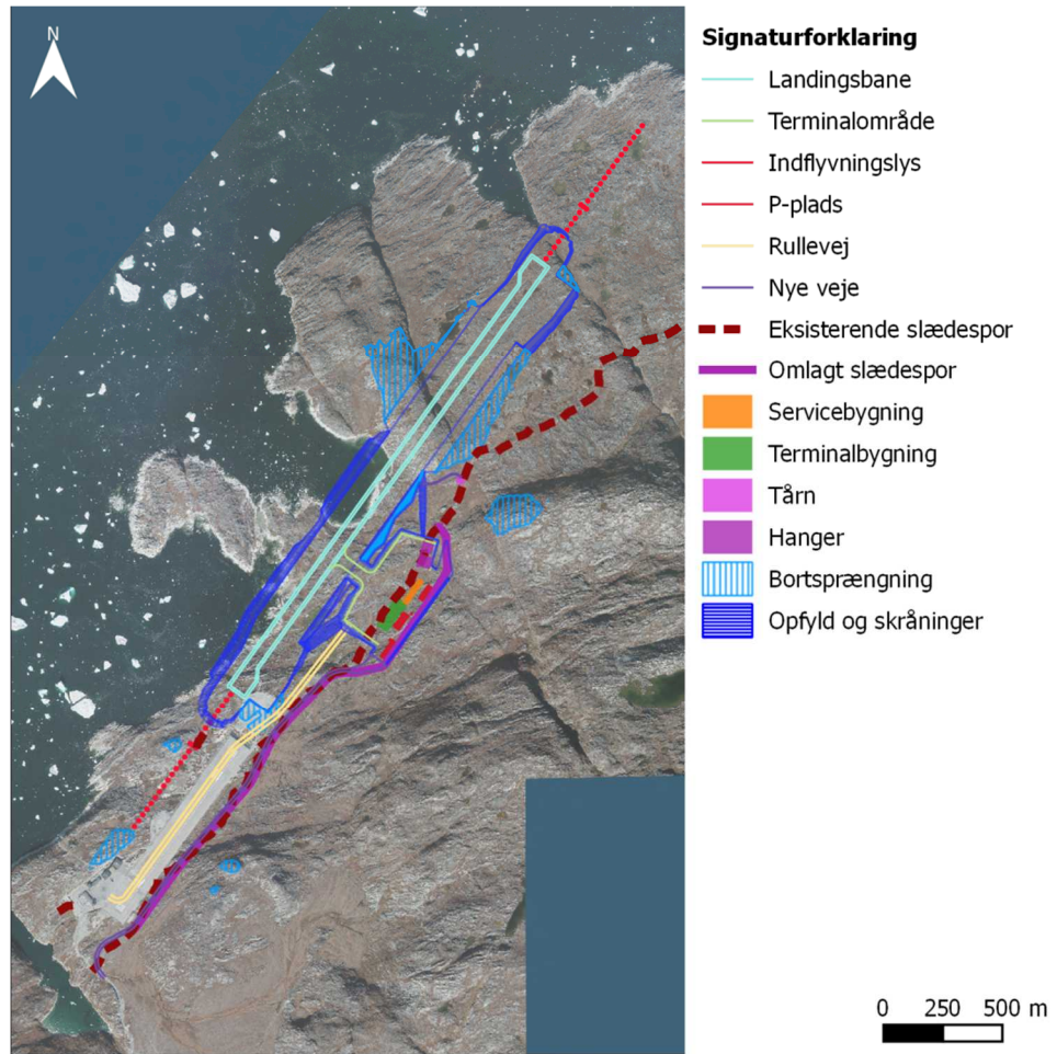
Takussutissiaq 3.11: Aqqusineq nutaamik sananeqarsimasoq kiisalu illerngit allangortinneqarsi- masut.
