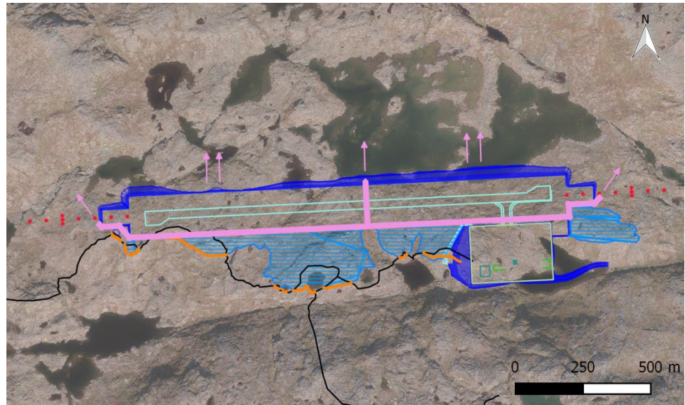
Takussutissiaq 3.7: Sumiifimmi paqqersaanerup ataqatigiineranik qalunaanit isiginnineq.
