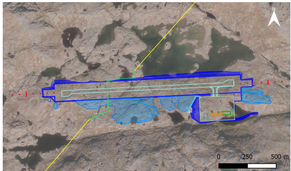
Takussutissiaq 3.5: Mittarfik kangimut-kimmut inissisimasoq.
