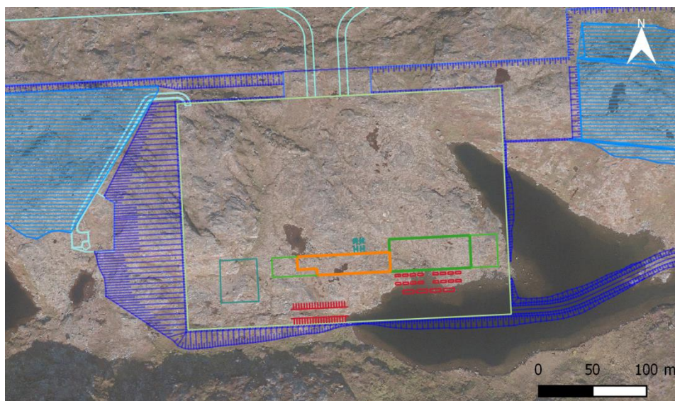
Takussutissiaq 3.6: Aallartarfittut tikittarfillu siunnersuutigineqartumik qulaanit isiginnineq.
